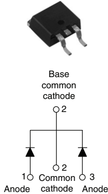
D 2 PAK
